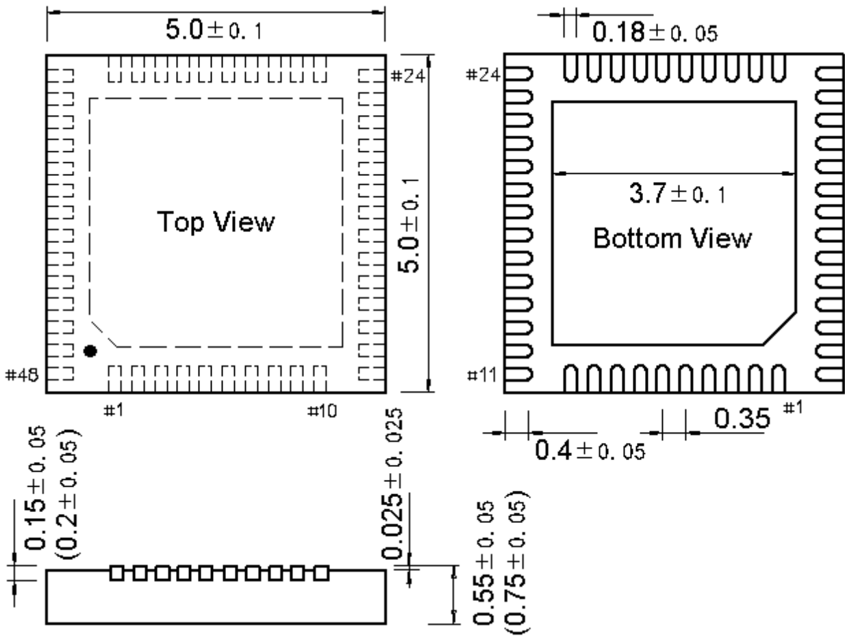
QFN48 (QFN48-5*5*0.55-0.35)
