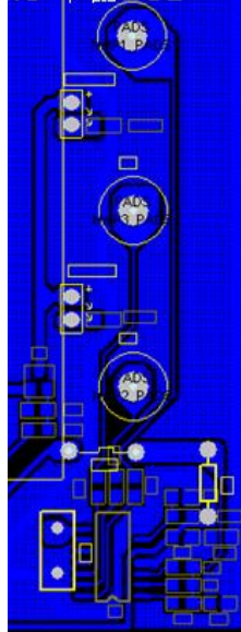
图 12: 采用单面 PCB 板, 弹簧作按键感应盘的 3 键电热水器触控板实例
