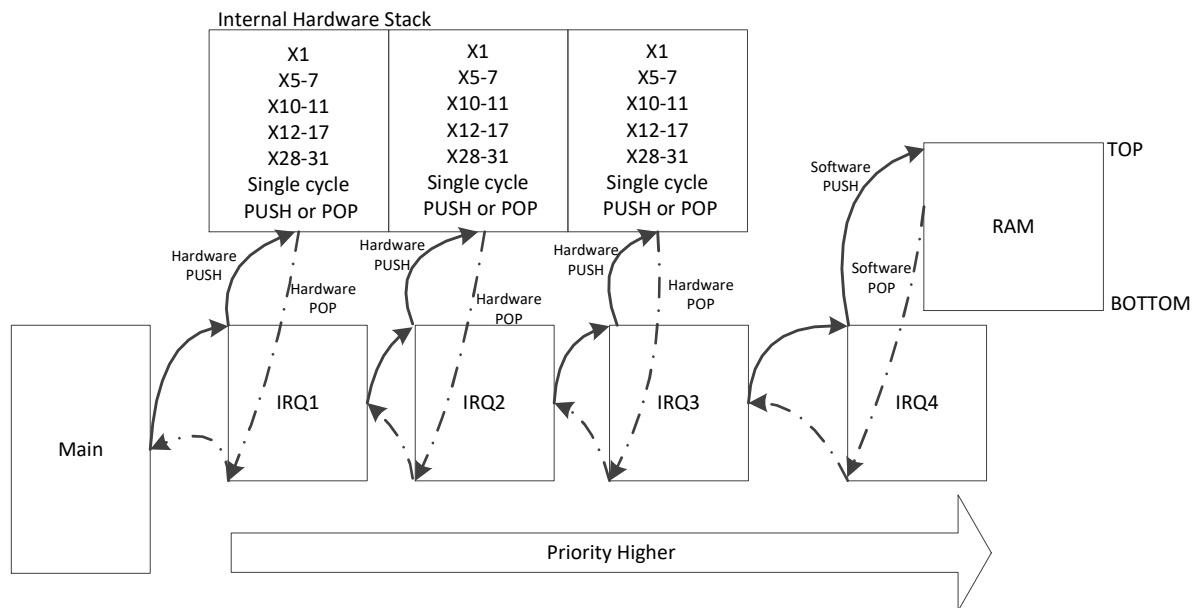
图 3-1 压栈示意图
